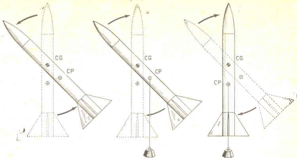
Fig. 4 - Dimostrazione pratica della funzione specifica di CG e CP. Un missile a stabilità positiva, nel caso una forza estranea intervenga a disturbare la rotta, tende ad inclinarsi ruotando su CG (a sinistra); le forze aerodinamiche agiscono su CP come se su detto fosse applicato un peso (al centro), costringendo il missile a ristabilizzarsi (a destra).
