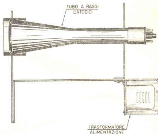
Fig. 9 - Il trasformatore di alimentazione deve risultare sistemato sotto il telaio, discosto — in altezza — il più possibile dallo zoccolo del tubo a raggi catodici. Tale accorgimento al fine di evitare che il campo magnetico creato dal trasformatore devii il fascio elettronico del tubo. Per una soluzione più radicale del problema, non mancheremo di schermare il tubo a raggi catodici.
