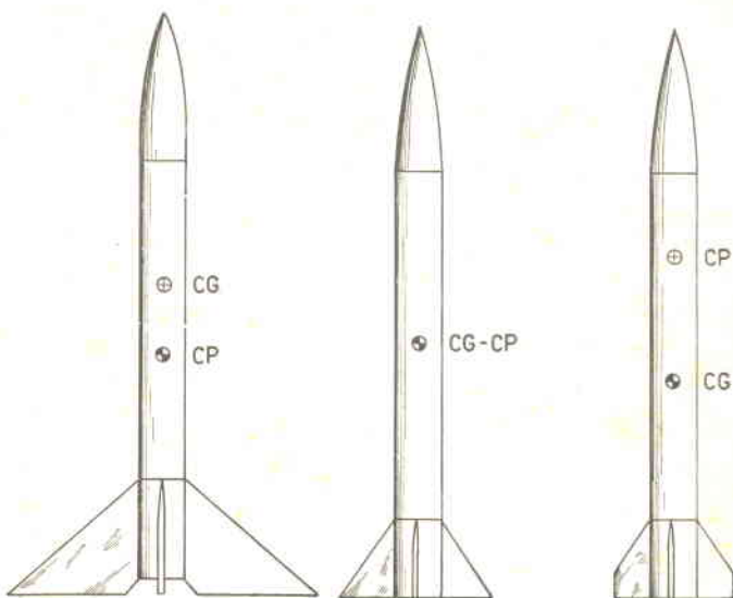
Fig. 3 - Oltre al CG, un missile presenta il Centro di Pressione. Al fine un missile presenti stabilità di volo, necessita che il CG risulti posto anteriormente al CP. A figura — a sinistra — un missile a stabilità positiva, cioè con caratteristiche di volo ottime. Al centro un missile a stabilità neutra, cioè non adatto ad essere lanciato per la pericolosità derivante. A destra un missile a stabilità negativa: il CG risulta posteriore a CP. In tal caso il missile, lasciata la rampa di lancio, volgerà l'ogiva verso terra.
