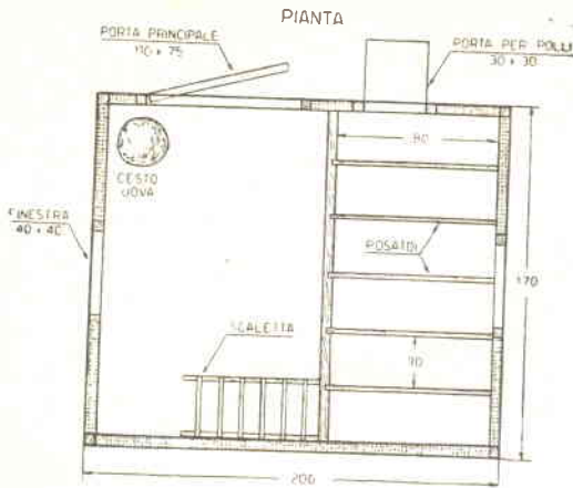
Fig. 5 - Pianta pollaio (dimensioni in centimetri).
