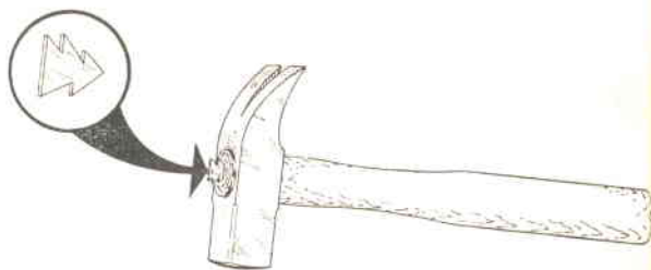
Fig. 2 - Nella costruzione dei manichi per martelli, necessita tener conto delle dimensioni della parte battente e regolarsi di conseguenza. Al fine di rendere solidale il martello al manico utilizzeremo un cuneo in ferro, lateralmente al quale solleveremo scaglie che impediranno lo sfilamento della parte battente.
