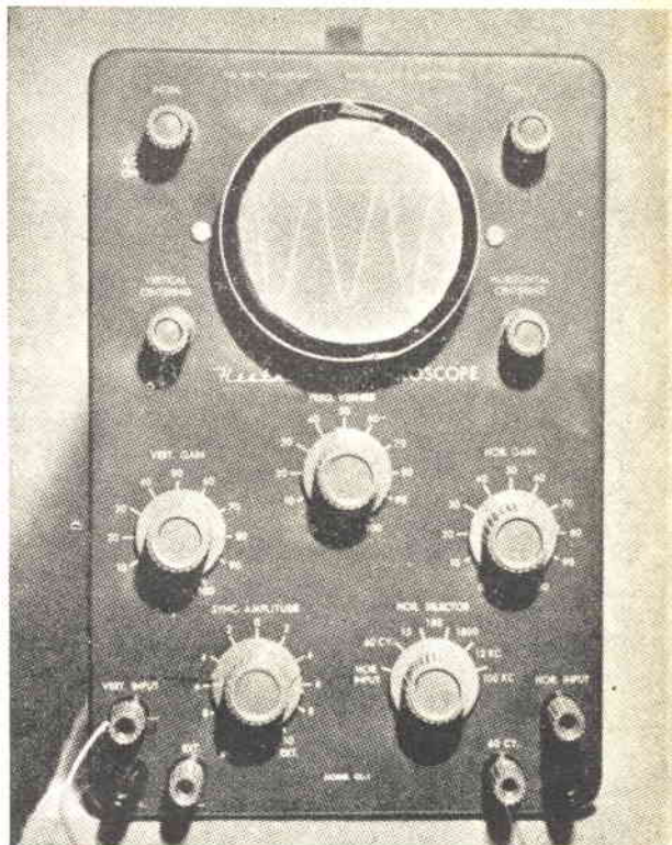
Fig. 1 Pannello frontale dell'oscilloscopio completo di comandi.
