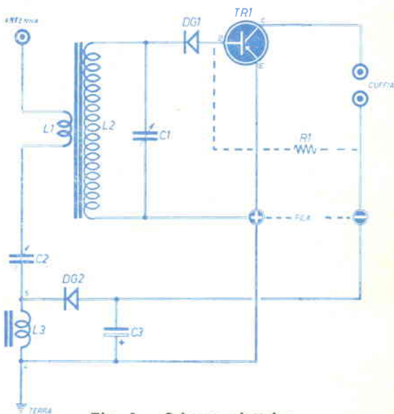
Fig. 1 - Schema elettrico.
