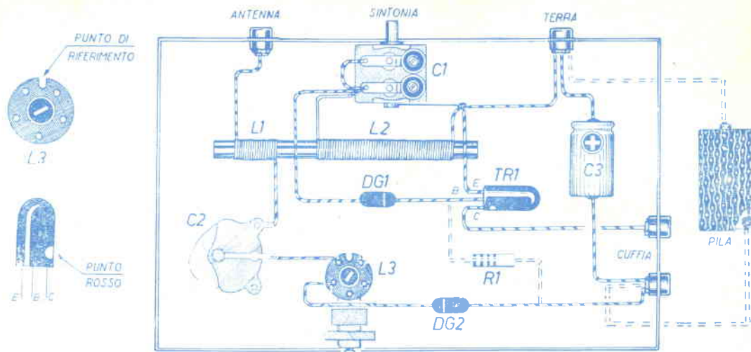
Fig. 2 - Schema pratico.
