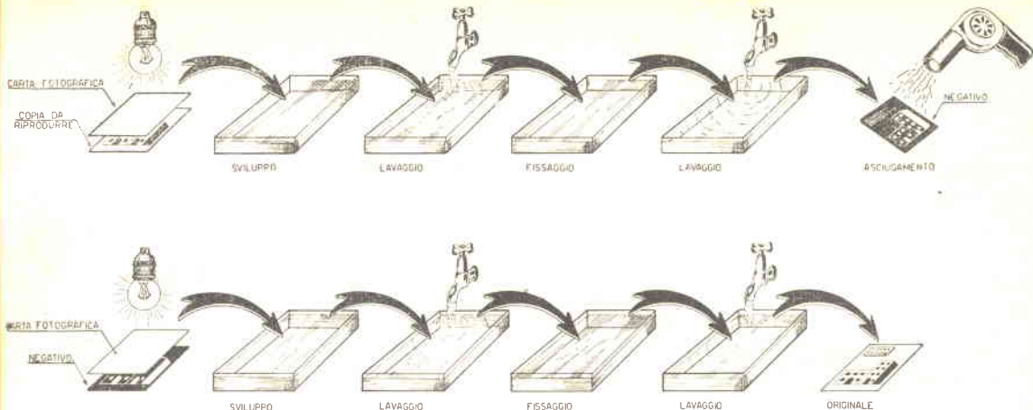
Fig. 6 - Dopo l'esposizione è necessario immergere la carta sensibile impressionata nel bagno di sviluppo (temperatura a 18° C.). Quando sulla carta risulteranno nitidi e neri i tratti, procederemo alla lavatura in acqua corrente, per poi immergerla — per 10 minuti — nel bagno di fissaggio. Lavata ancora e riasciugata la copia, saremo in possesso di un negativo, che utilizzeremo — seguendo procedimento analogo a quello usato precedentemente — per la realizzazione di copie dell'originale.
