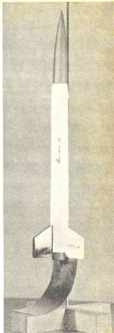
Fig. 9 - Si rivela necessario che il missile risulti guidato — in partenza — per un metro almeno, sì che al momento del distacco dalla base di lancio il medesimo si ritrovi in possesso della velocità necessaria all'autostabilizzazione. Infatti, similmente ad una freccia scoccata da un arco poco teso, se la velocità di partenza risulterà ridotta, il missile punterà l'ogiva verso terra dopo breve volo.
