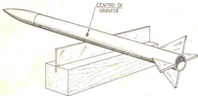
Fig. 8 - Il centro di gravità CG lo si rintraccerà a missile completato, ricercandone la posizione di equilibrio sul taglio di una lama. Per distanziare CG da CP risulterà sufficiente o aumentare il peso dell'ogiva, o aumentare la superficie delle alette.
