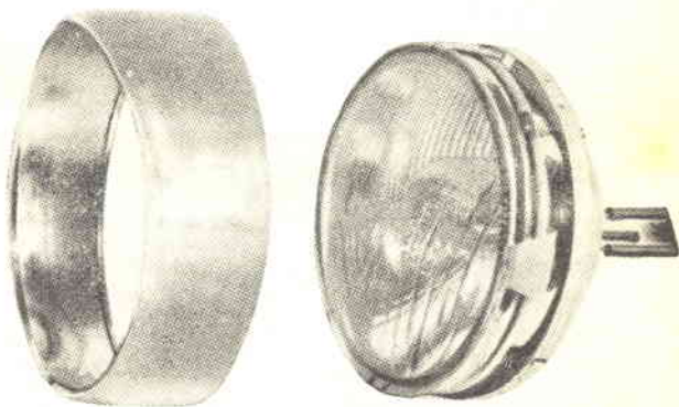
Fig. 1 - In certi casi riuscirà utile, anziché procedere alla sola sostituzione del gruppo ottico, montare — in luogo del normale in dotazione — un proiettore asimmetrico di diametro maggiore. Tale sostituzione presenta il vantaggio di notevolmente accrescere il volume di luce a disposizione.
