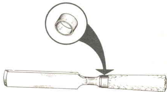
Fig. 3 - Ad evitare che il manico abbia a muoversi, si consiglia — qualora risulti possibile — cingerne la sommità con un anello in metallo, ottenibile da spezzone di tubo di dimensioni idonee. L'anello — ovviamente — verrà inserito prima dell'introduzione nel manico del codolo dell'utensile.
