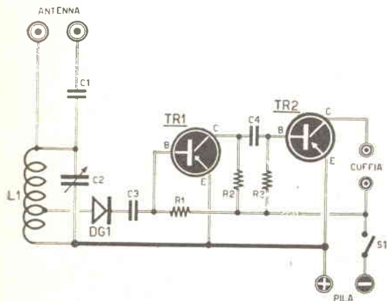
SCHEMA ELETTRICO
