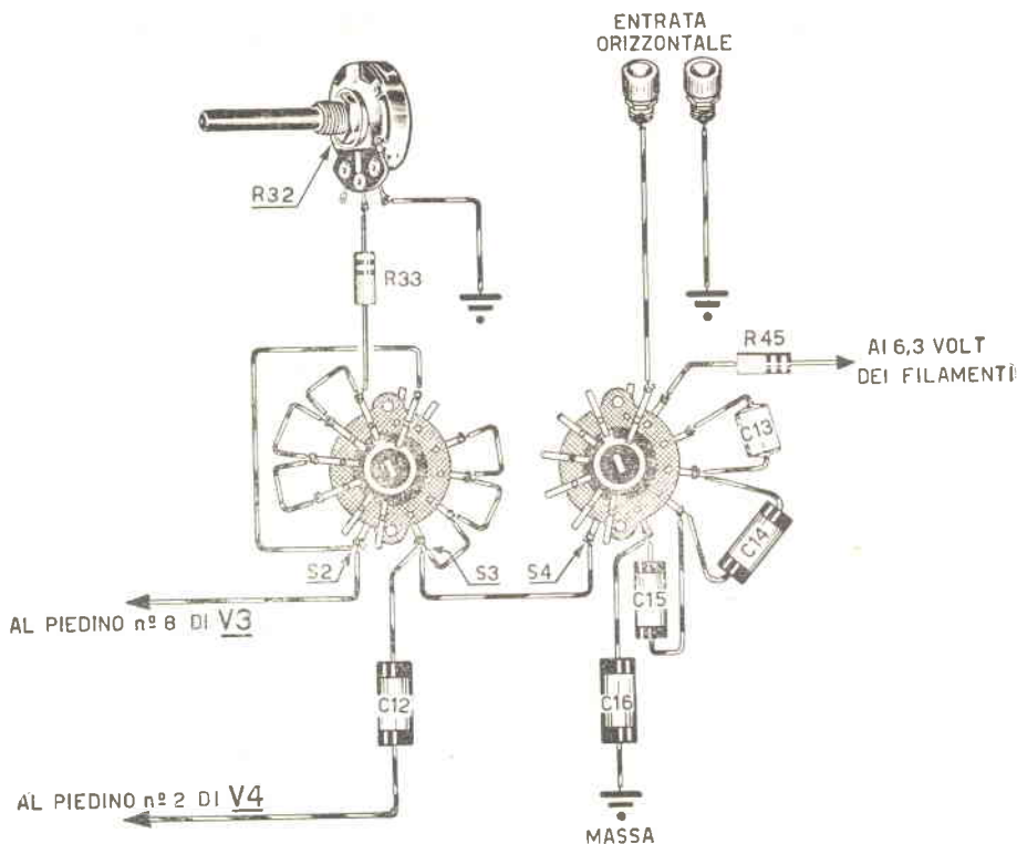
Fig. 10 - S2 - S3 - S4 costituiscono unico commutatore a 6 posizioni 4 vie (serve egregiamente il Geloso N. 20222 di catalogo). Per i meno esperti indicammo il collegamento dei vari terminali del commutatore. Precisiamo che una delle 4 vie del commutatore — precisamente quella abbinata a S4 — rimane inoperosa.
