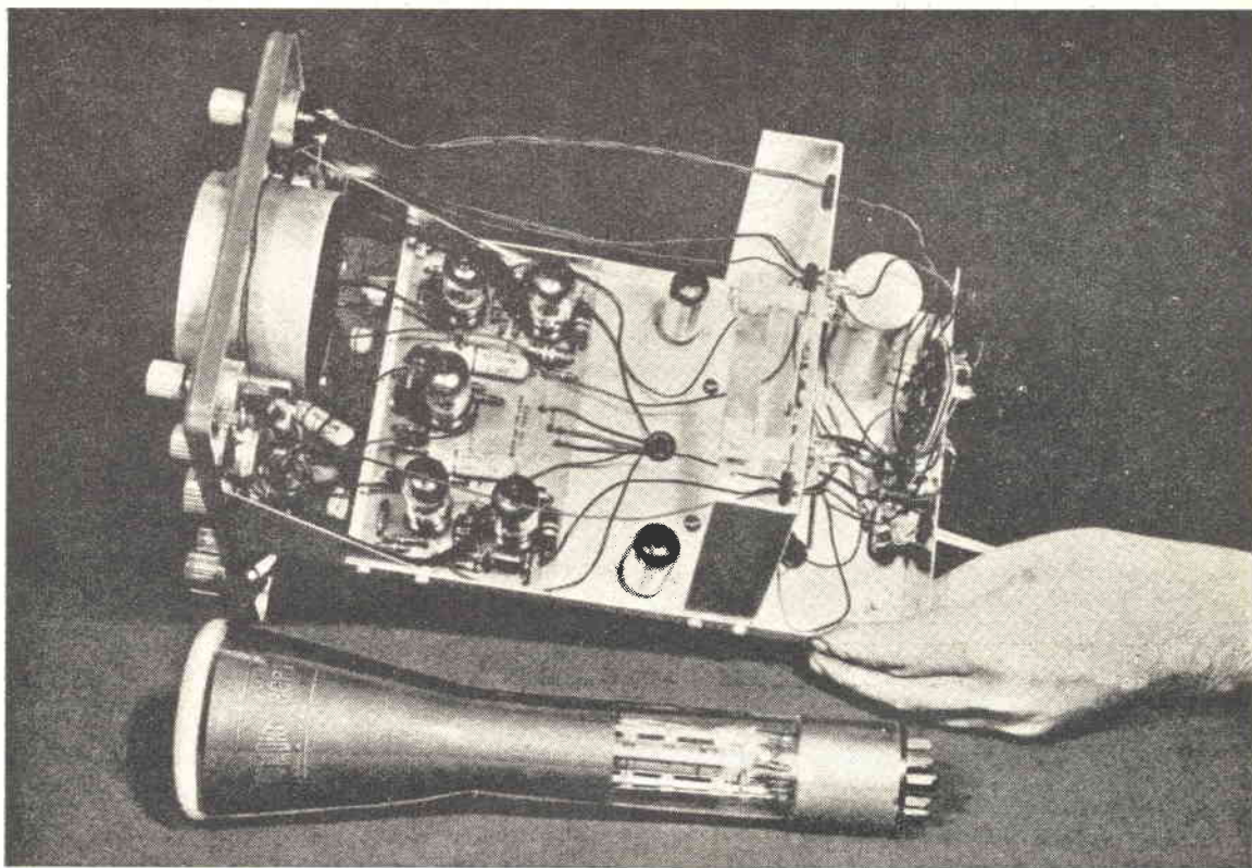
Fig. 3 - L'oscilloscopio visto dall'alto. Si noti la disposizione delle valvole e la posizione del supporto tubo a raggi catodici. Detto supporto, che risulta assicurato al pannello, oltre che svolgere funzioni di sostegno del tubo, funge pure da paralucente.
