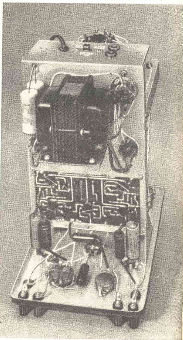
Fig. 6 - Il trasformatore di alimentazione, ad evitare dannose influenze dovute al campo magnetico creato, verrà sistemato inferiormente al telaio. Si consiglia pure la messa in opera di un trasformatore blindato.
