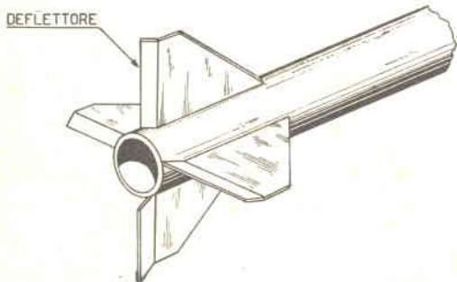
Fig. 6 - Per conferire maggior stabilità al missile si potrà tentare di dotare il medesimo di moto rotativo attorno al suo asse longitudinale. Ciò potrà conseguirsi con l'applicazione alle estremità delle pinne di deflettori. Adottando tal sistema non saremo in grado però di far raggiungere al missile considerevoli altezze.
