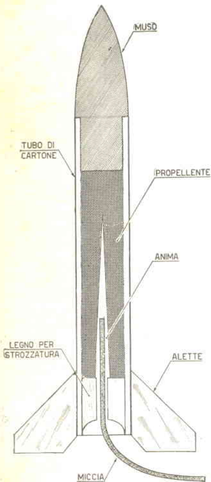
Fig. 10 - La carica con polvere nera verrà effettuata prevedendo un'anima tronco-conica, al fine di conseguire una più vasta superficie di accensione e conseguenziale maggior produzione di gas, condizione basilare per imprimere al missile una elevata velocità. La carica verrà accesa sempre a mezzo miccia. Il foro del tappo in legno risulterà 8 volte minore del diametro del missile.
