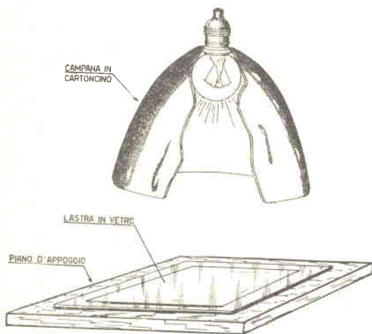
Fig. 4 - Per rendere uniforme la luce sulla carta sensibile, costruiremo una campana in cartoncino bianco, la cui circonferenza di bordo venga a coprire interamente la superficie del documento da riprodurre.
