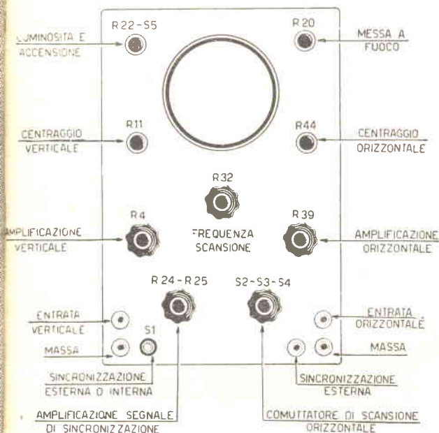
Fig. 7 - Disposizione comandi sul pannello frontale.
