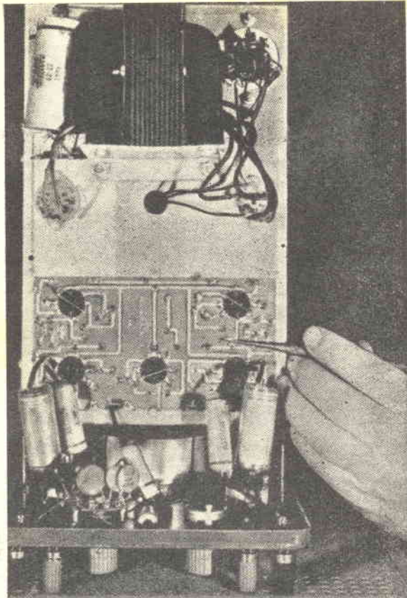
Fig. 5 - Nel caso dello stadio amplificatore sarà possibile utilizzare pure circuiti stampati, come è dato vedere a foto.
