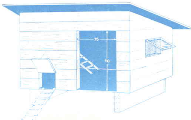
Fig. 3 - Porta di pulizia e apertura accesso-uscita polli
