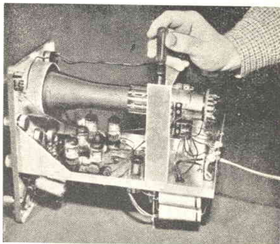
Fig. 4 - L'oscilloscopio montato.
