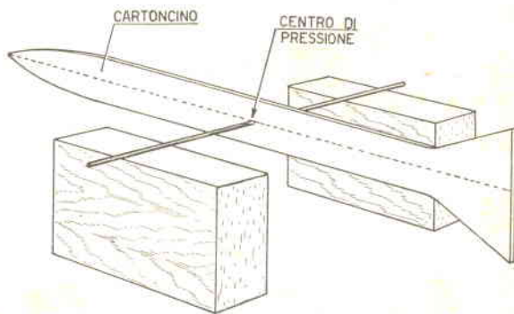
Fig. 7 - Il centro di pressione CP si rintraccerà ritagliando una sagoma in cartoncino rigido del missile visto di lato e ricercandone il punto di equilibrio.
